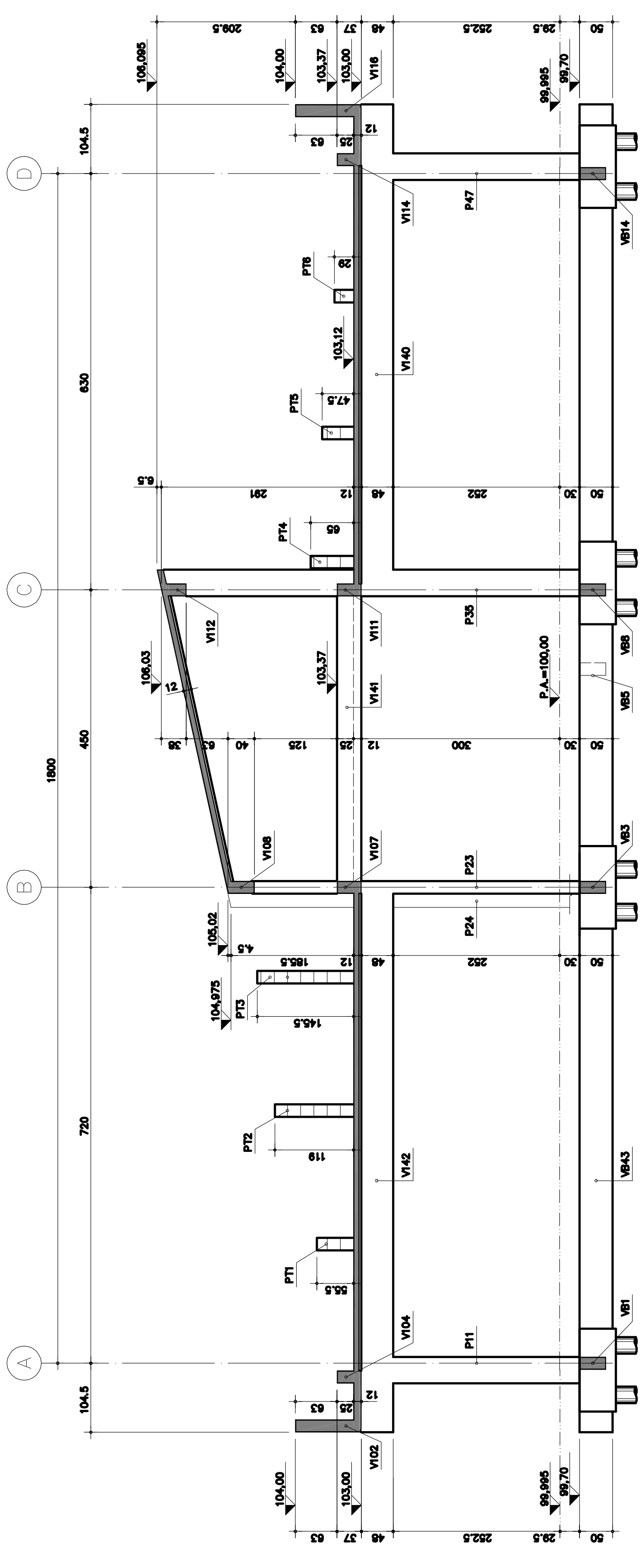
CORTE B-B ESC. 1:50
